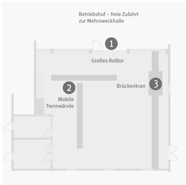
Grundriss Mehrzweckhalle
