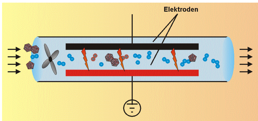
Abbildung Schematische Darstellung eines NTP- Reaktors
